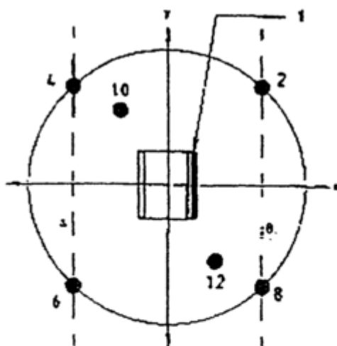
Figura 39.2 Dettaglio della struttura e del montaggio del percorso di scorrimento
