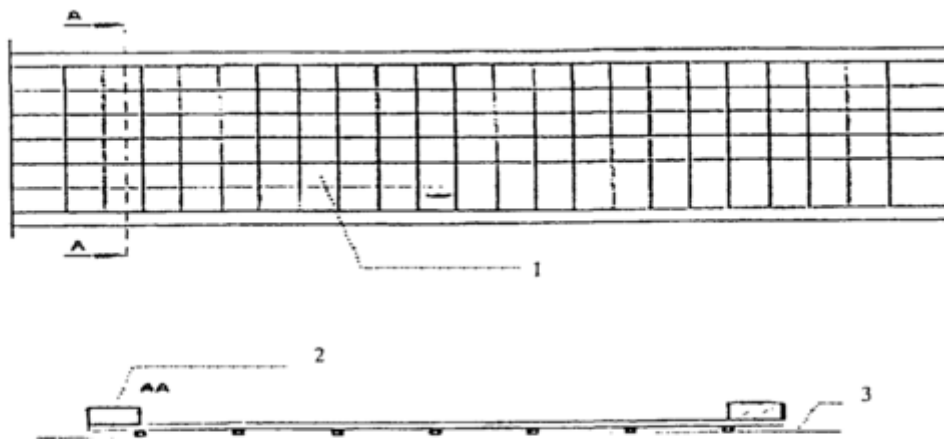
Figura 39.1 : Disegno del percorso di scorrimento
