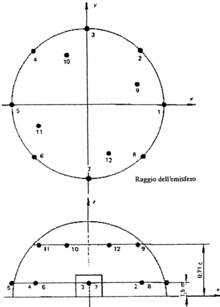
Posizionamento dei microfoni supplementari sull'emisfero (12 posizioni)
